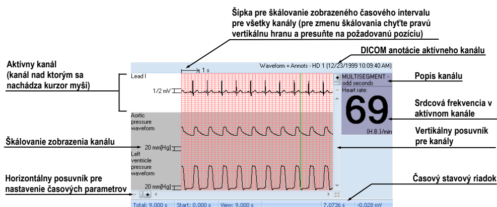
obr. 385 – Náhľadové okno pre diagnostiku EKG/HD kriviek
