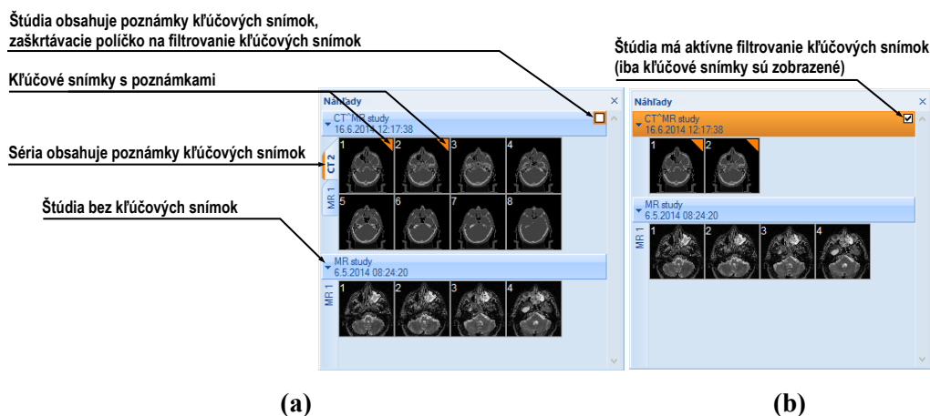
obr. 174 – Poznámky kľúčových snímok v palete náhľadov, (a) filtrovanie pre kľúčové snímky je neaktívne, (b) filtrovanie pre kľúčové snímky je aktívne
