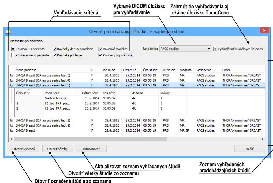
obr. 110 – Dialóg Otvorenie predchádzajúcich štúdií
