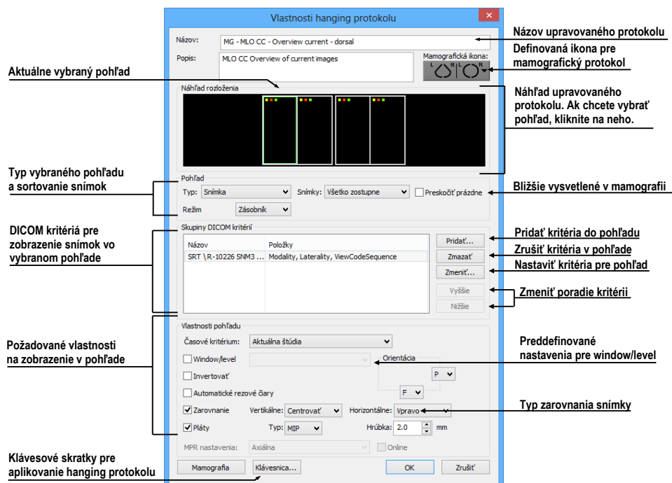
obr. 188 – Dialóg Vlastnosti hanging protokolu
