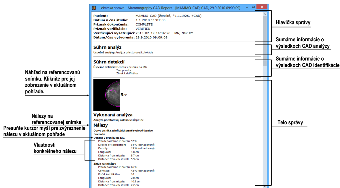
obr. 401 – Náhľad Mammo CAD správy
