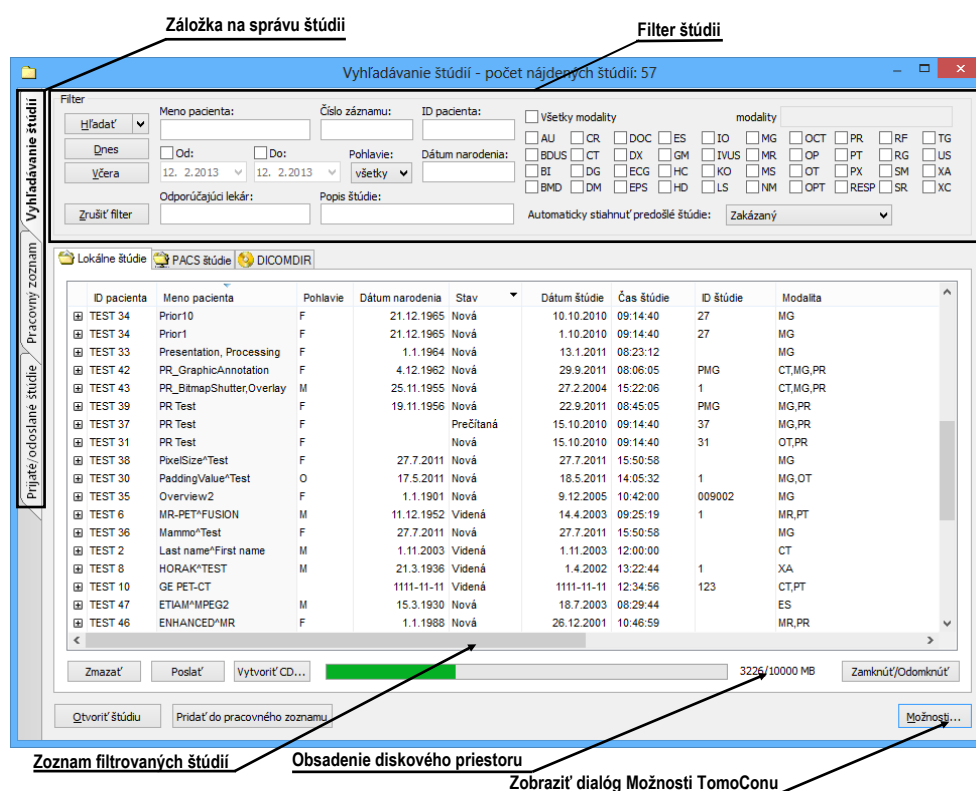
obr. 86– Hlavné časti dialógu Vyhľadávanie štúdií
