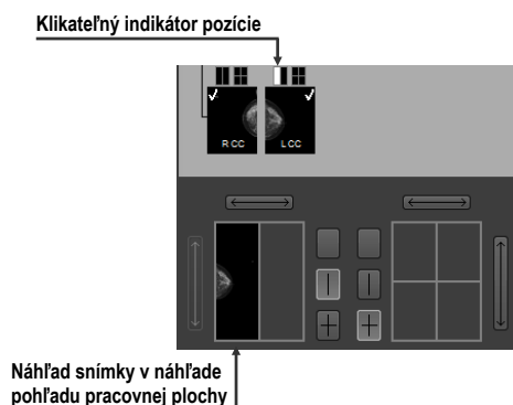
obr. 458 – Kliknite na obdĺžnik v indikátore pre zobrazenie alebo skrytie snímky v príslušnom pohľade
