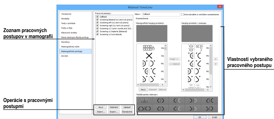
obr. 449 – Záložka Mamografické postupy
