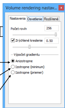
obr. 321 – Volume rendering nastavenia, prvá záložka
