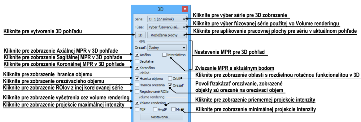
obr. 277 – Nástrojový dialóg 3D
