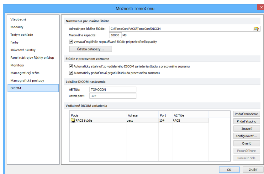
obr. 75 – Záložka DICOM dialógu Možnosti TomoConu
