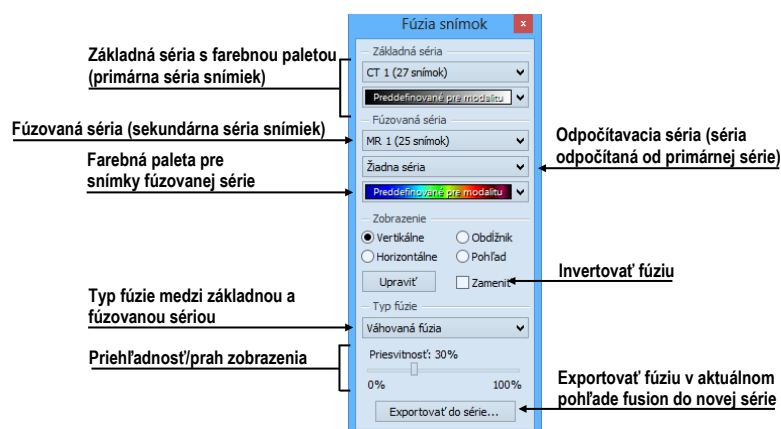
obr. 270 – Nástrojový dialóg Fúzia
