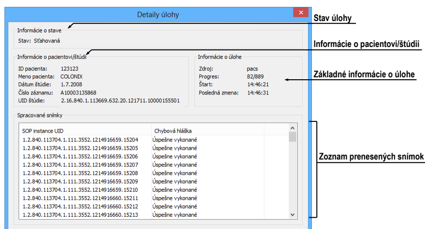
obr. 114 – Dialóg Detaily úlohy
