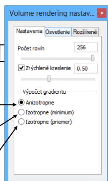
obr. 288 – Volume rendering nastavenia, prvá záložka
