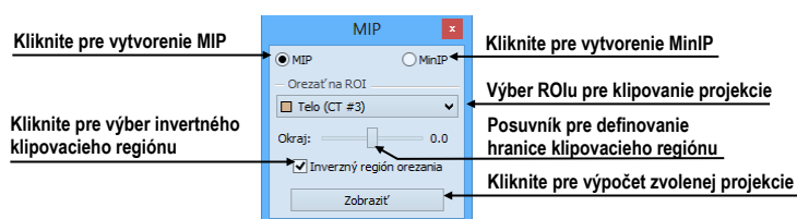
obr. 267 – Nástrojový dialóg MIP/minIP
