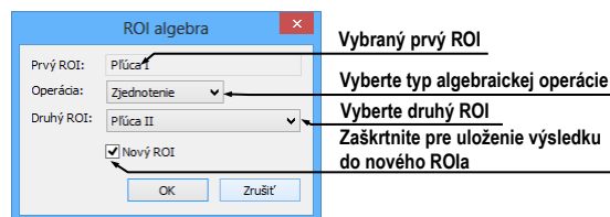
obr. 236 – ROI Algebra dialóg
