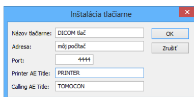
obr. 325 – Dialóg Inštalácia tlačiarne
