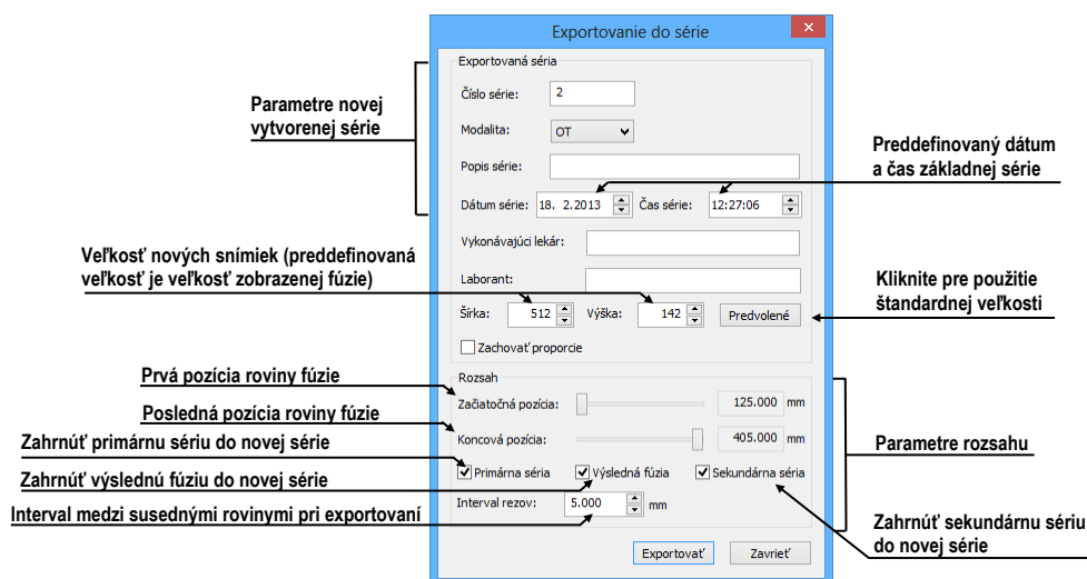
obr. 276 - Dialóg Exportovanie do série (parametre novej série)
