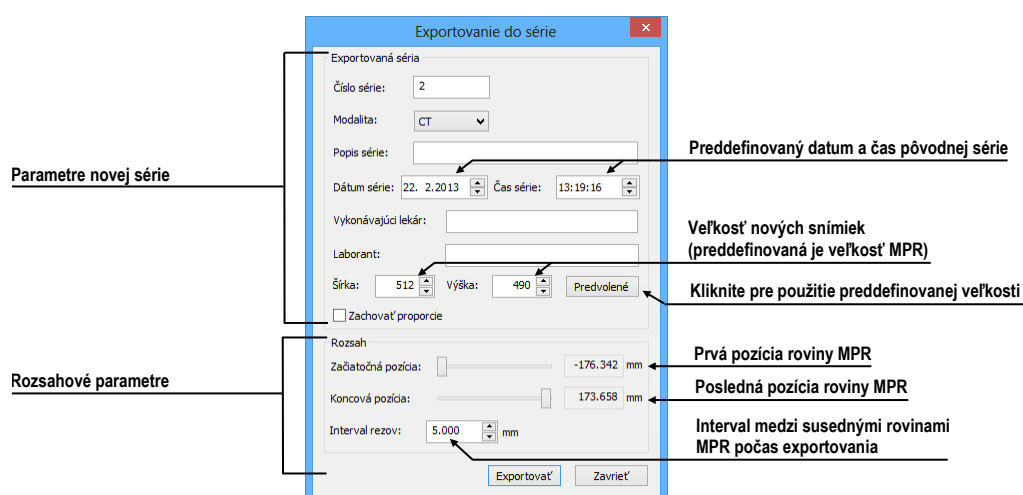
obr. 266 – Dialóg Exportovanie do série
