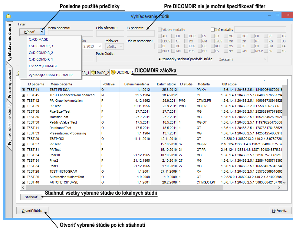
obr. 100 – DICOMDIR v dialógu Vyhľadanie štúdií
