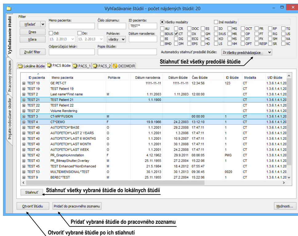
obr. 99 – Výber štúdií na PACS serveri
