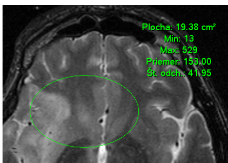
obr. 203 – Elipsa
