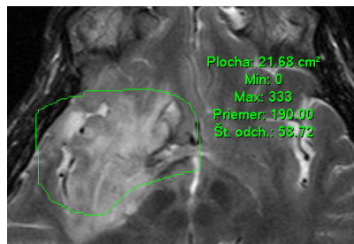
obr. 207 – Všeobecná plocha
